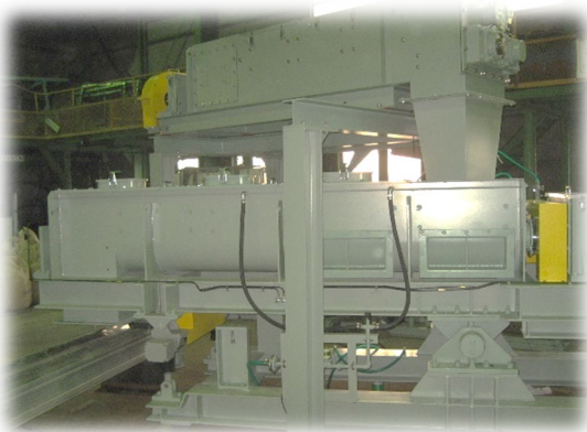
混練機と造粒機
